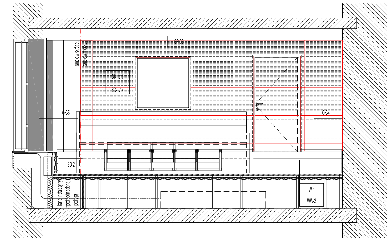
WIDOK ŚCIANY 4-4
